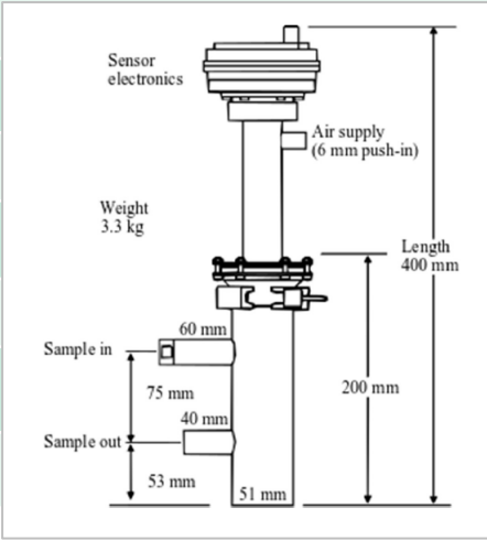
PPS-M寸法
