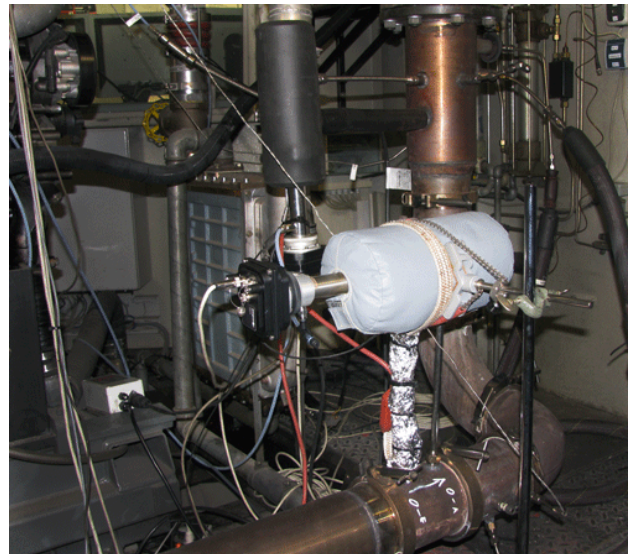
エンジンベンチ接続例
