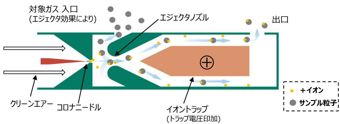
センサー内部構造図
