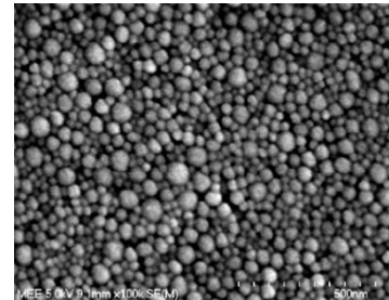
SEMによるシリカのスラリー写真
