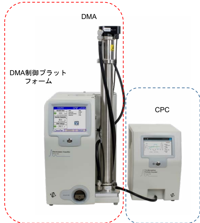
DMA(静電分級器) CPC(凝縮粒子カウンター)
