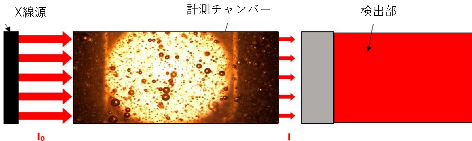
X線透過による密度測定
