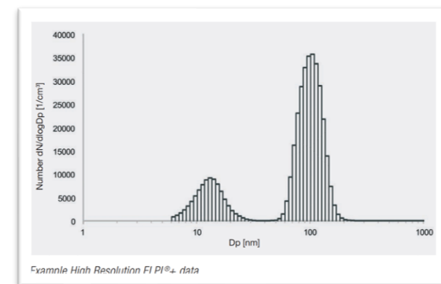
HR-ELPI+粒径グラフィイメージ
